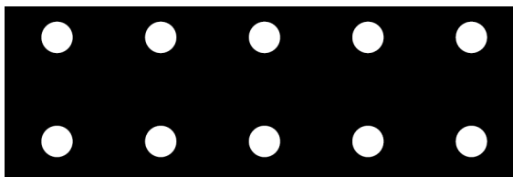
RG 4,5/15,0; a_o = 7,1\%
